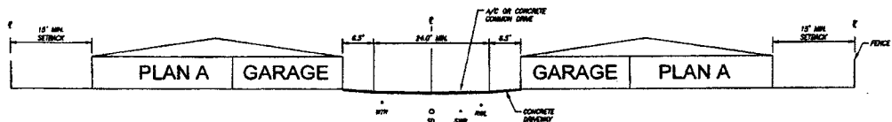
SECTION A-A
